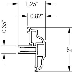
22 EXTERIOR LITE FRAME ODL
